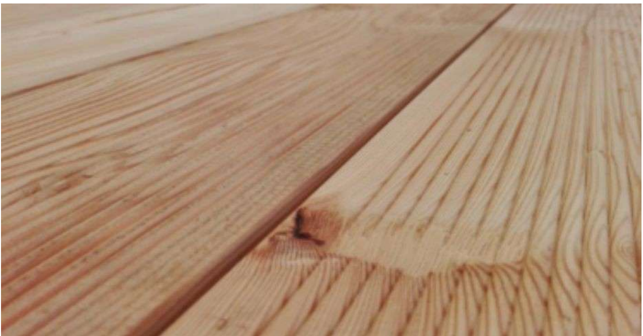
Foto 24 – ein beim Hobeln herausgerissener Teil
